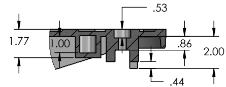
Detalle T Escala 1 : 6
