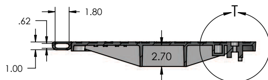
Sección B-B
