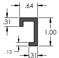
Junta de Goma (Material - Neopreno)
