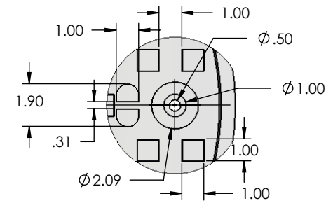
Detalle X Escala 1 : 6
