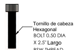
Perno de bloqueo (Material - Acero Inoxidable)
