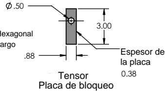
Detalle T Escala 1 : 6
