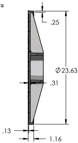
Sección A-A
