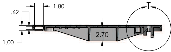
Sección B-B
