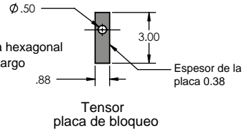
Detalle T Escala 1 : 6
