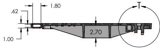
Sección B-B
